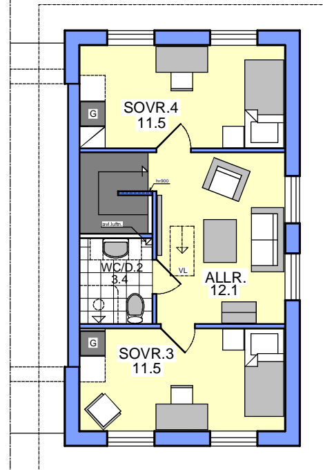
ÖVRE PLAN BOA 43.2 m 2
