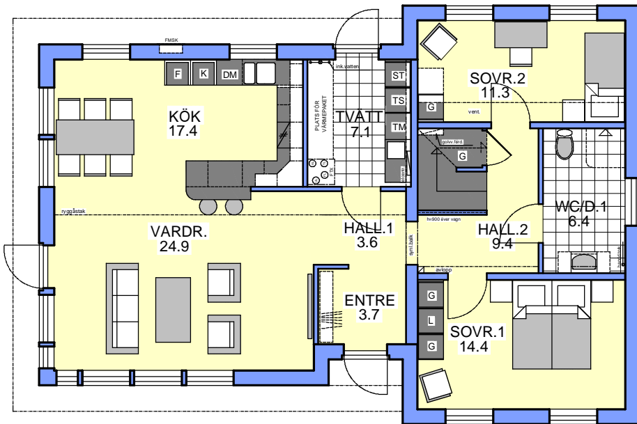
ENTRÉPLAN BOA 102.2 m 2 TOT BOA 145.4 m 2
